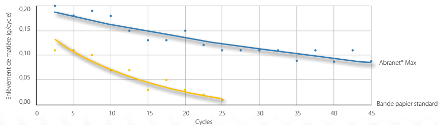
Abranet® Max vs bande papier standard P120 – Ponçage de chêne
